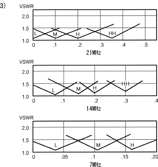
714XW VSWR (代表例)
